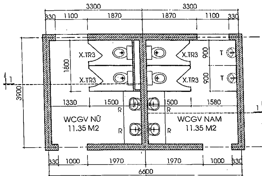
MẶT BẰNG
