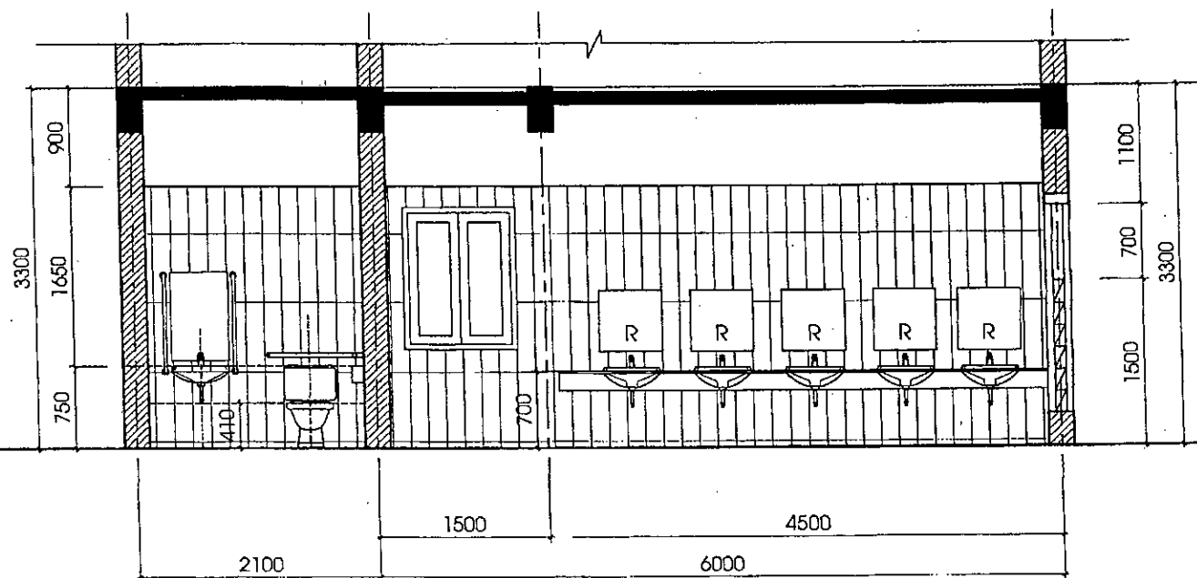
MẶT CẮT 1-1
