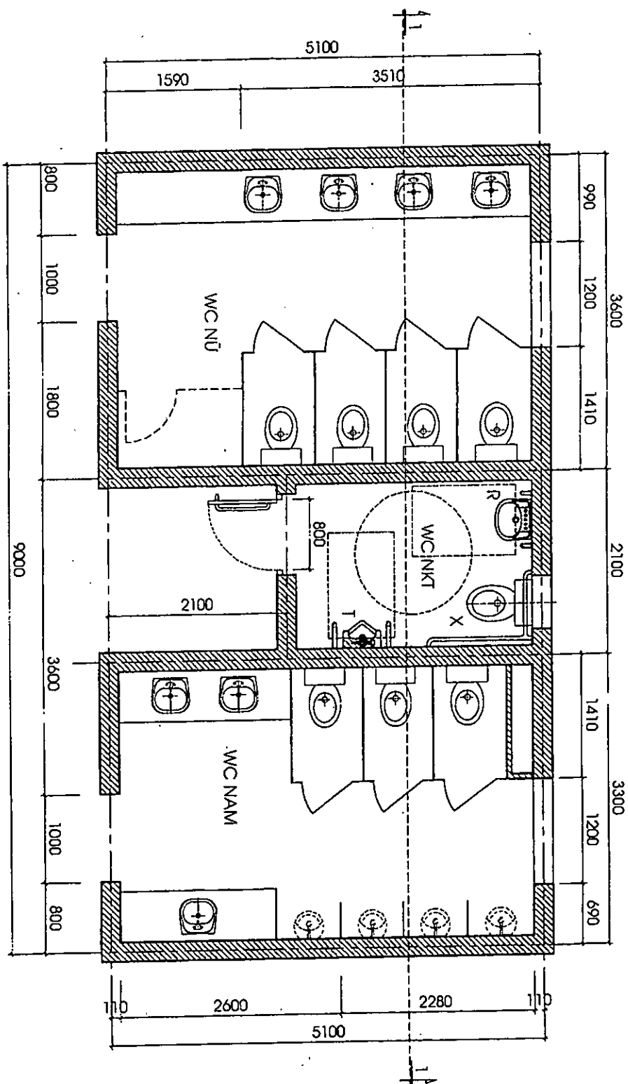
MẶT BẰNG
