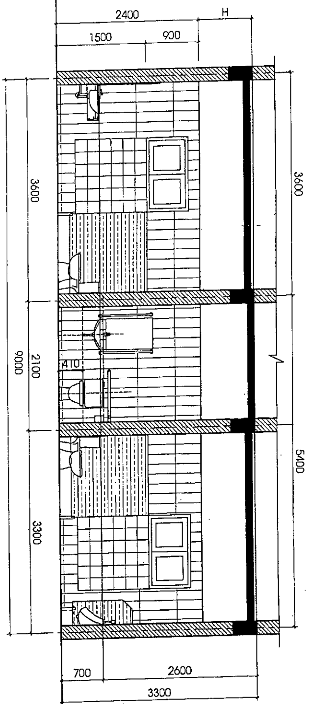
MẶT CẮT 1-1
