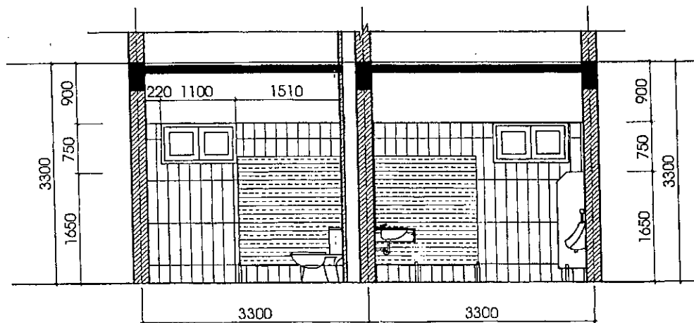
MẶT CẮT 1-1
